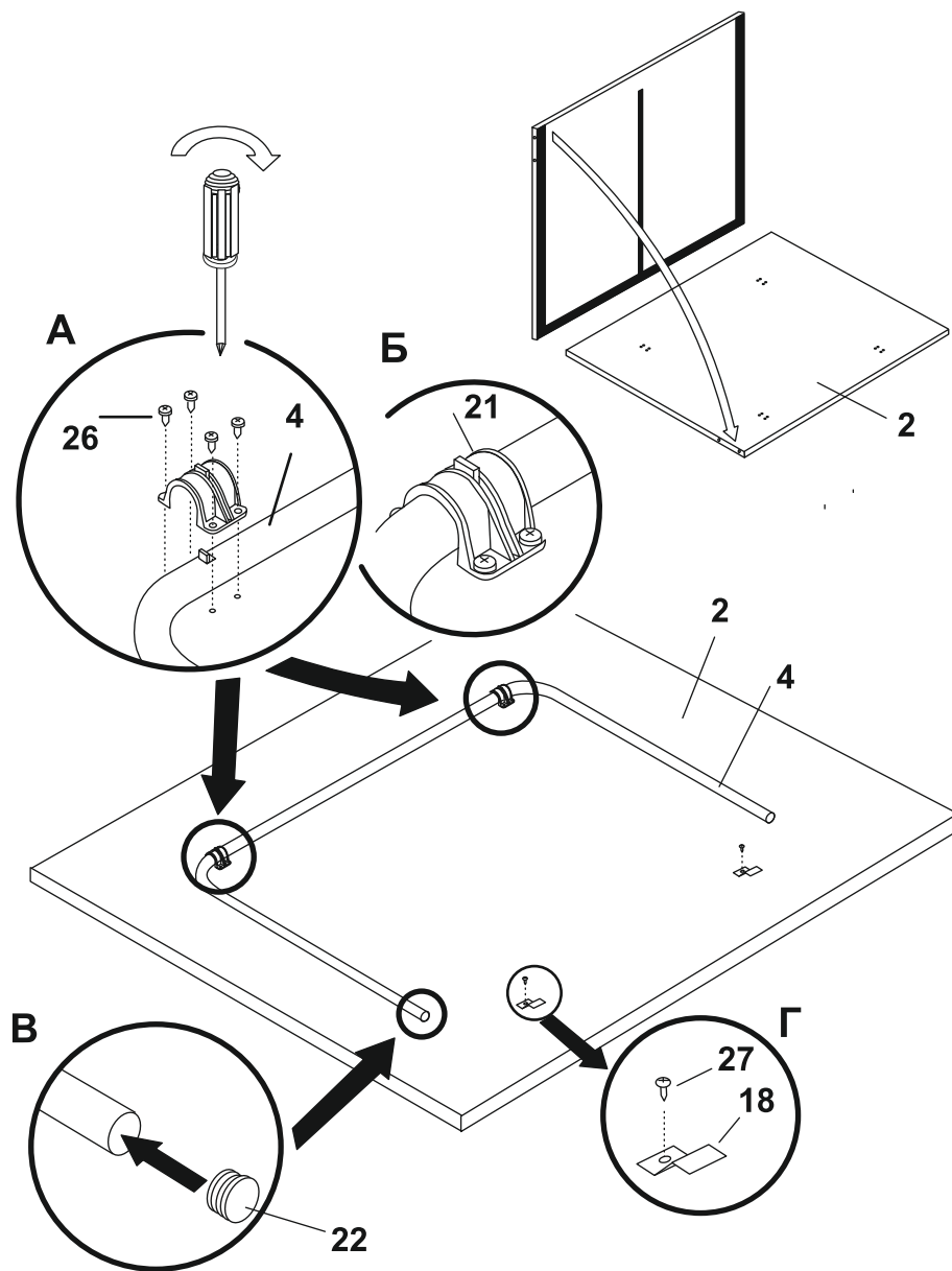
Сборка столешницы. Рис. 4
