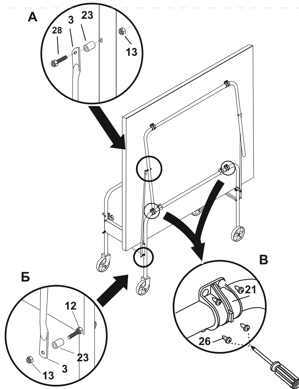
Установка столешницы на каркас (Рис. 5)
